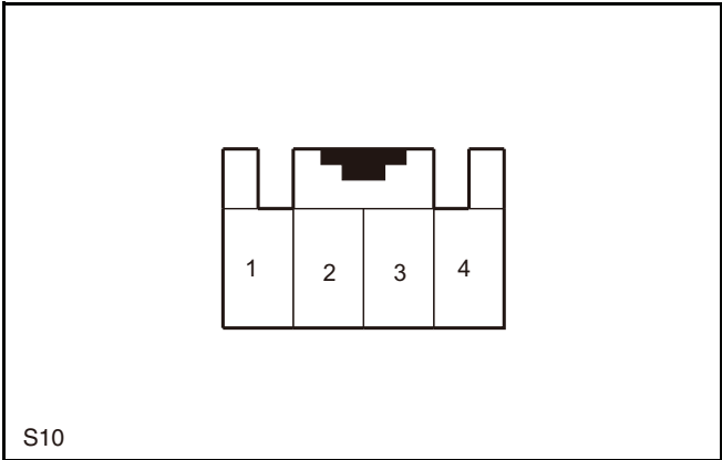
S10 驾驶员座椅加热控制器
