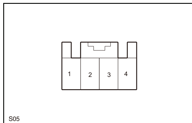
S05 乘客座椅加热控制器
