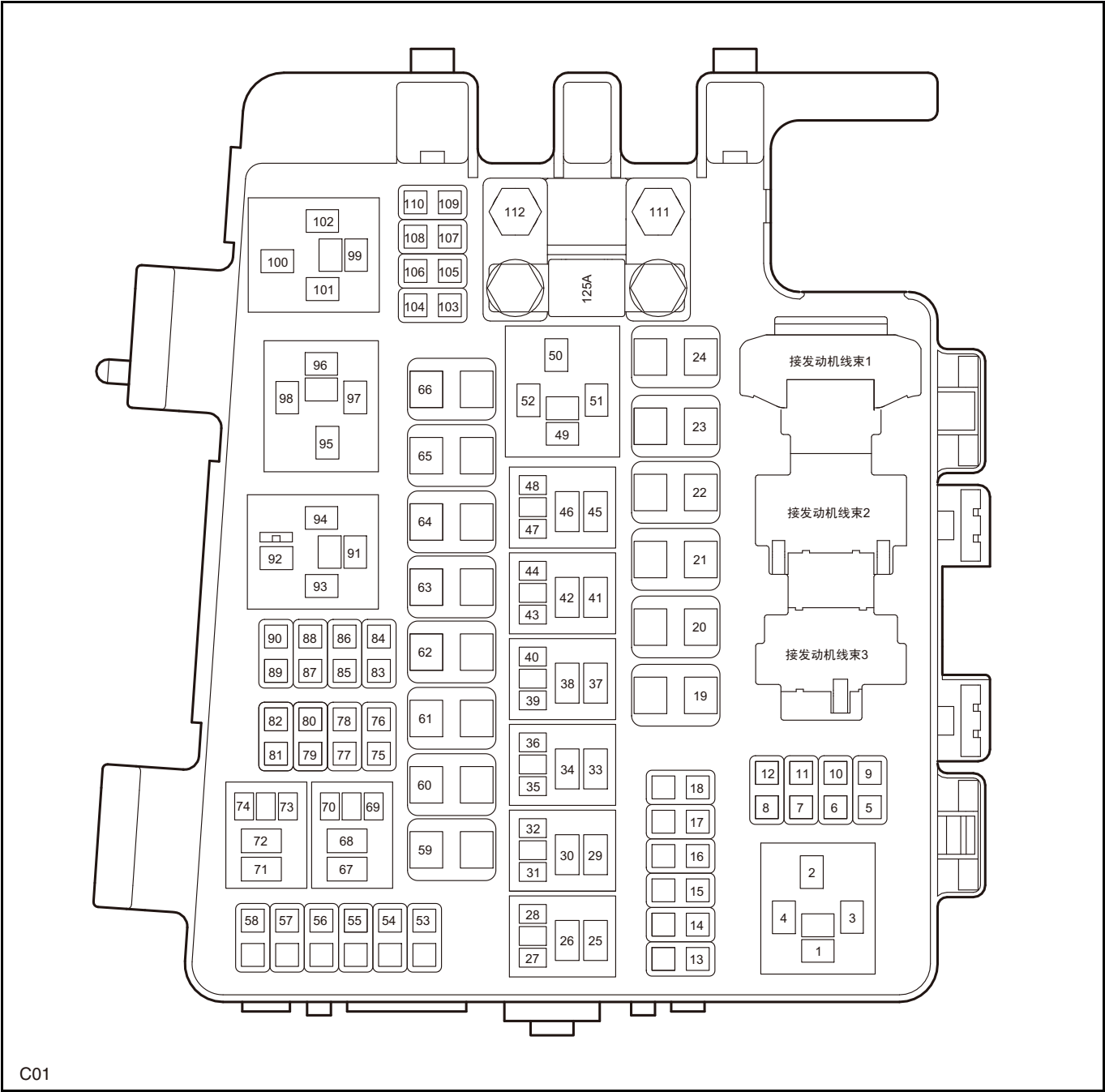
C01 发动机舱电器中心
