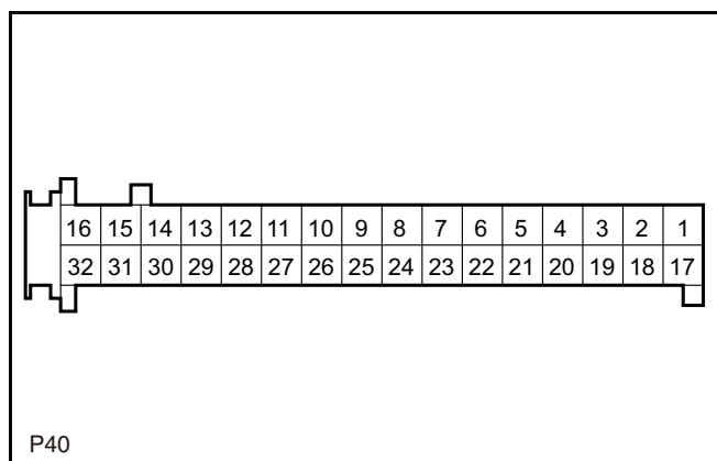
P40 自动空调控制器
